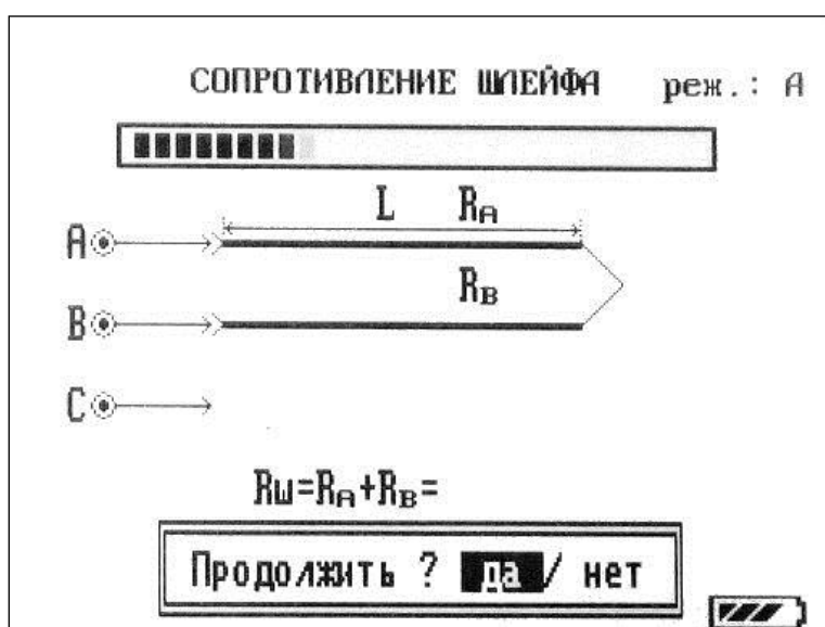
Рисунок 6-15 Измерение сопротивления шлейфа
