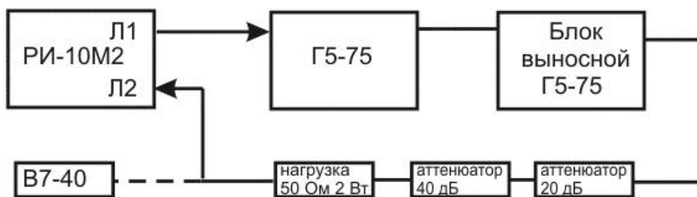
Рисунок 9-8 Схема определения чувствительности приёмного тракта
