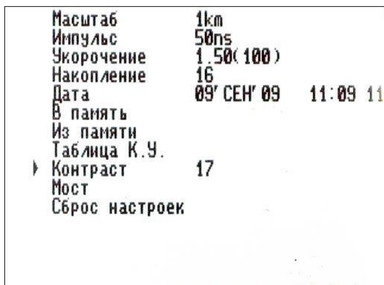
Рисунок 4-3 Вид дисплея в режиме МЕНЮ рефлектометра
