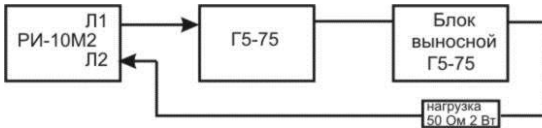
Рисунок 9-5 Схема поверки диапазона измерений расстояния (временной задержки)
