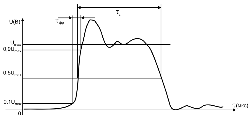
Рисунок 9-7 Форма зондирующего импульса
