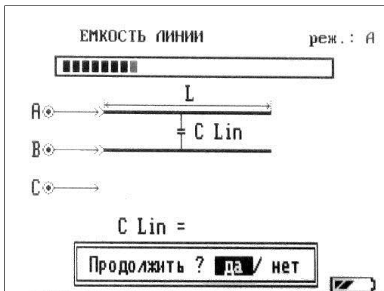
Рисунок 6-17 Измерение ёмкости линии
