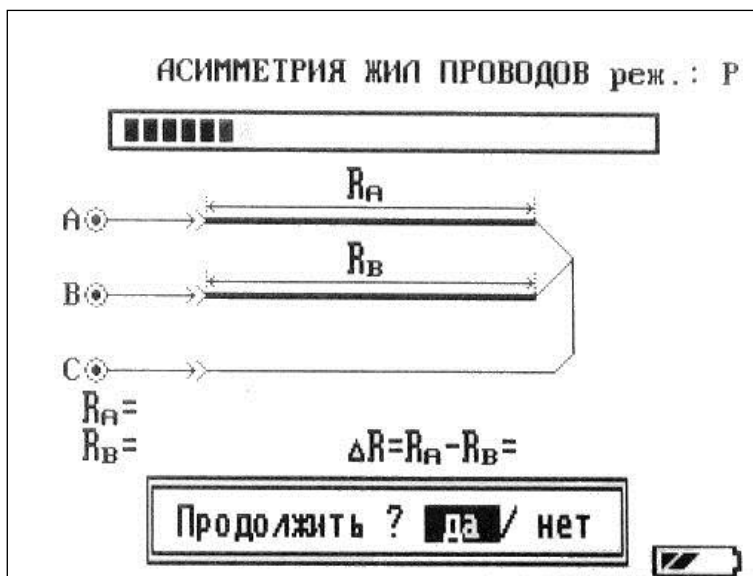
Рисунок 6-16 Измерение асимметрии жил проводов
